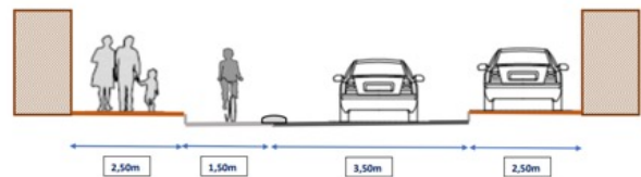
COUPE EN TRAVERS DE L'AMENAGEMENT PROJETE
